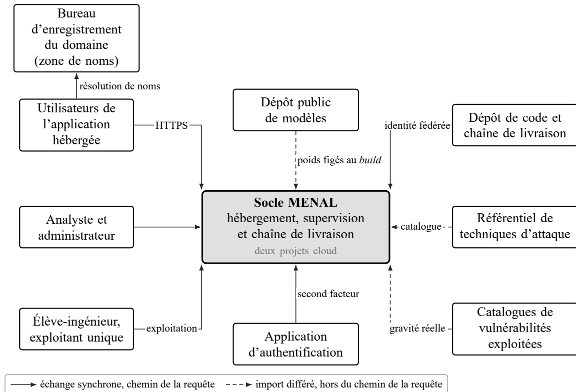
FIG. 9. Vue de contexte : le socle, ses acteurs et les six systèmes extérieurs dont il dépend — trois imports différés portent le risque de chaîne d’approvisionnement, la zone de noms échappe seule à la description en code (É10)
