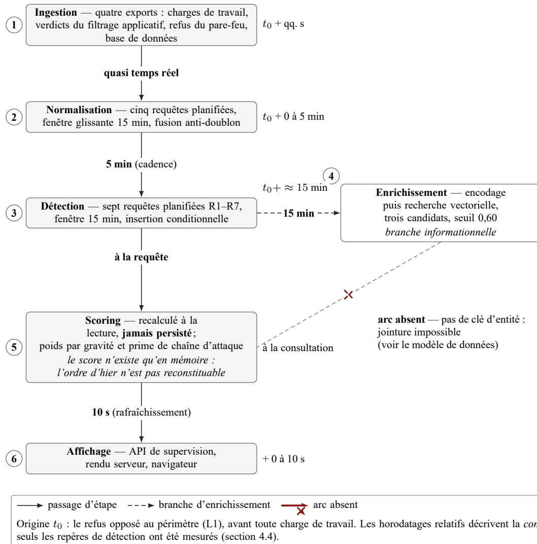
FIG. 14. Cycle de vie de la donnée de sécurité : six étapes, le budget de latence porté par les cadences et l'horodatage relatif de chaque étape. Le délai entre l'événement et son affichage est fait d'attentes d'ordonnanceur et non de temps de traitement : trois attentes s'additionnent (5 + 5 + 15 min), et aucune puissance de calcul ne les réduirait. La branche d'enrichissement n'alimente pas le calcul de score — impasse fonctionnelle assumée.
