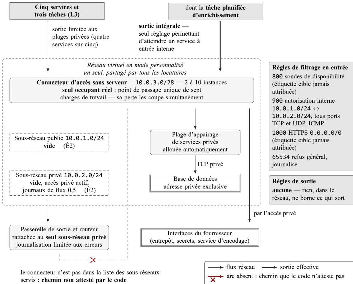
FIG. 12. Topologie réseau avant la refonte — état du dépôt jusqu'au 11/08/2026. La sortie des charges de travail n'y était pas gouvernée par le réseau mais par le paramètre de la plateforme d'exécution : la passerelle ne desservait que le sous-réseau privé, lequel était vide, et la plage qui portait la totalité de la sortie ne lui était pas rattachée. Aucune règle de sortie n'existait : c'est le diagnostic qui a motivé D15.
