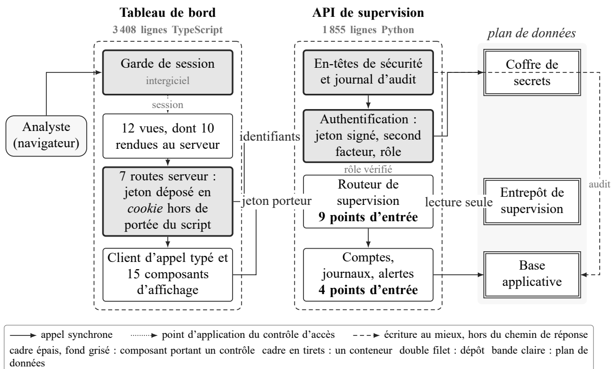
FIG. 23. Architecture interne des deux logiciels écrits : composants, frontières de déploiement et points d'application du contrôle d'accès. Le rôle est vérifié sur les treize points d'entrée de données de l'API — neuf de supervision et quatre de gestion — et jamais dans le tableau de bord, qui ne détient aucune autorisation propre ; l'échec de l'écriture d'audit est absorbé et ne fait jamais échouer la requête de l'analyste.
