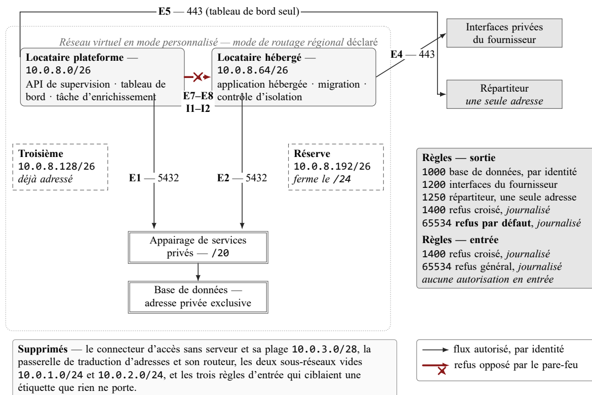
FIG. 13. Topologie réseau après la refonte appliquée du 11 au 25/08/2026 — le réseau en service à 25/08/2026, à comparer à la figure 12. Les charges de travail émettent depuis un sous-réseau : le pare-feu leur est applicable, et aucune autorisation ne comporte de plage source.
