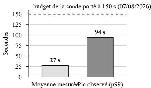
FIG. 30. Démarrage à froid du service d’encodage : moyenne et pic mesurés début août 2026, comparés au budget de la sonde de disponibilité.
