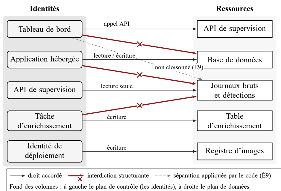
FIG. 17. Plan d'identité : droits accordés et interdictions structurantes (cinq identités). Ni l'application hébergée ni la tâche d'enrichissement ne peuvent écrire sur les preuves (scénario SO16, test T11); le tableau de bord passe par l'API de supervision, mais son identité conserve un droit de lecture sur l'entrepôt — c'est l'écart É9.
