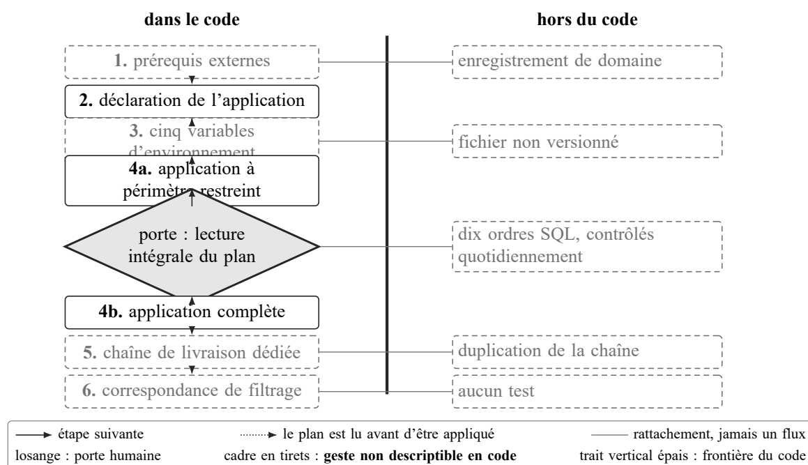
FIG. 26. Accueil d'un locataire : six étapes, et les cinq gestes qui restent hors du code. L'accueil est reproductible sur le plan de l'identité et du déploiement ; les cinq gestes non descriptibles en code sont la mesure exacte de la maturité multi-locataire du socle.
