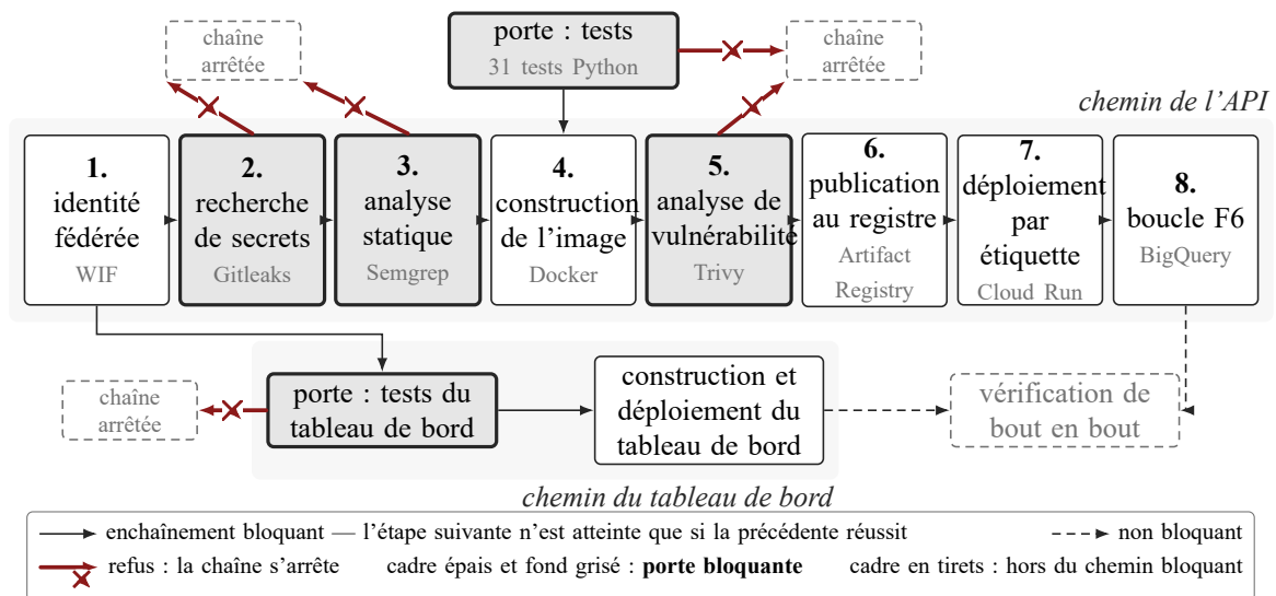
FIG. 21. Chaîne de livraison applicative. Chemin de l'API : huit étapes, dont trois portes bloquantes, plus la porte de tests qui conditionne la construction ; chemin du tableau de bord : sa propre porte. La vérification de bout en bout suit le déploiement et ne le défait pas — c'est une vérification, non une porte. Les cas de refus sont décrits en section 5.2.6 ; deux d'entre eux portent un protocole numéroté, T8 et T10, dont le chapitre 6 donne le verdict daté.
