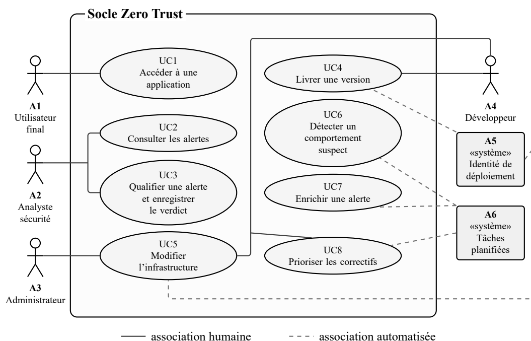
FIG. 7. Diagramme de cas d'utilisation du socle
