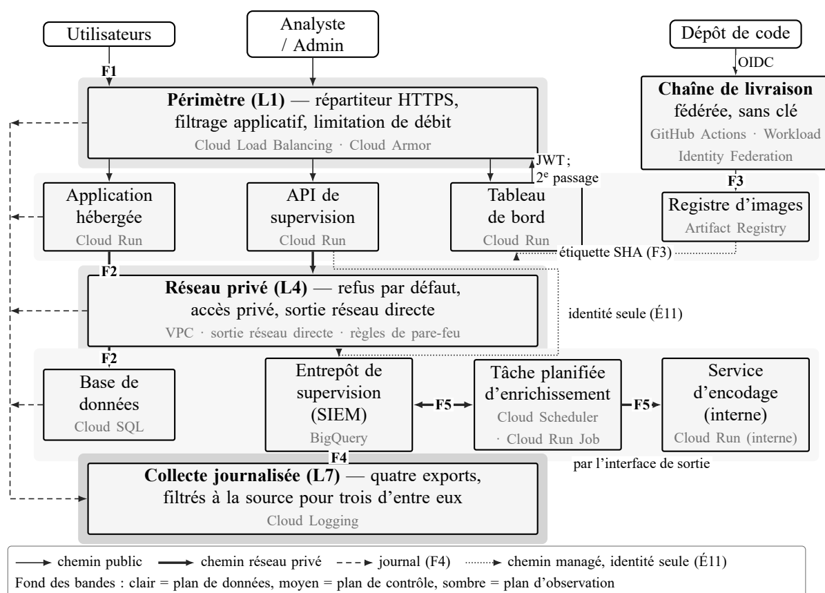
FIG. 11. Vue de déploiement : composants, liens réseau et flux F1 à F5. Le tableau de bord n'atteint les données que par l'API, et son appel ressort par le répartiteur : il subit un second passage du filtrage applicatif.
