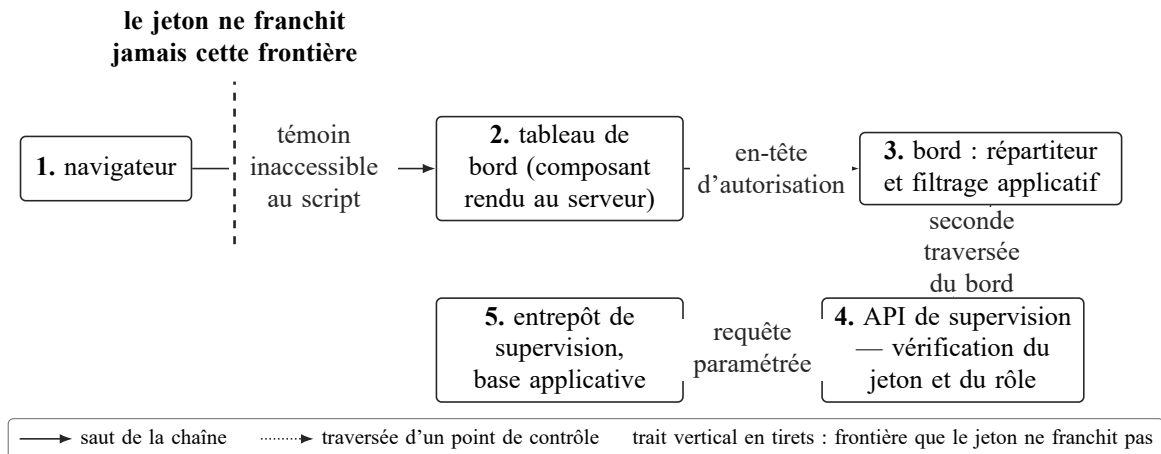
FIG. 24. Chaîne de données d'une vue du tableau de bord : les cinq sauts, et la frontière que le jeton ne franchit pas. L'autorité d'autorisation est l'API de supervision, qui vérifie le jeton et le rôle; l'identité du tableau de bord ne détient aucune autorisation sur les données.
