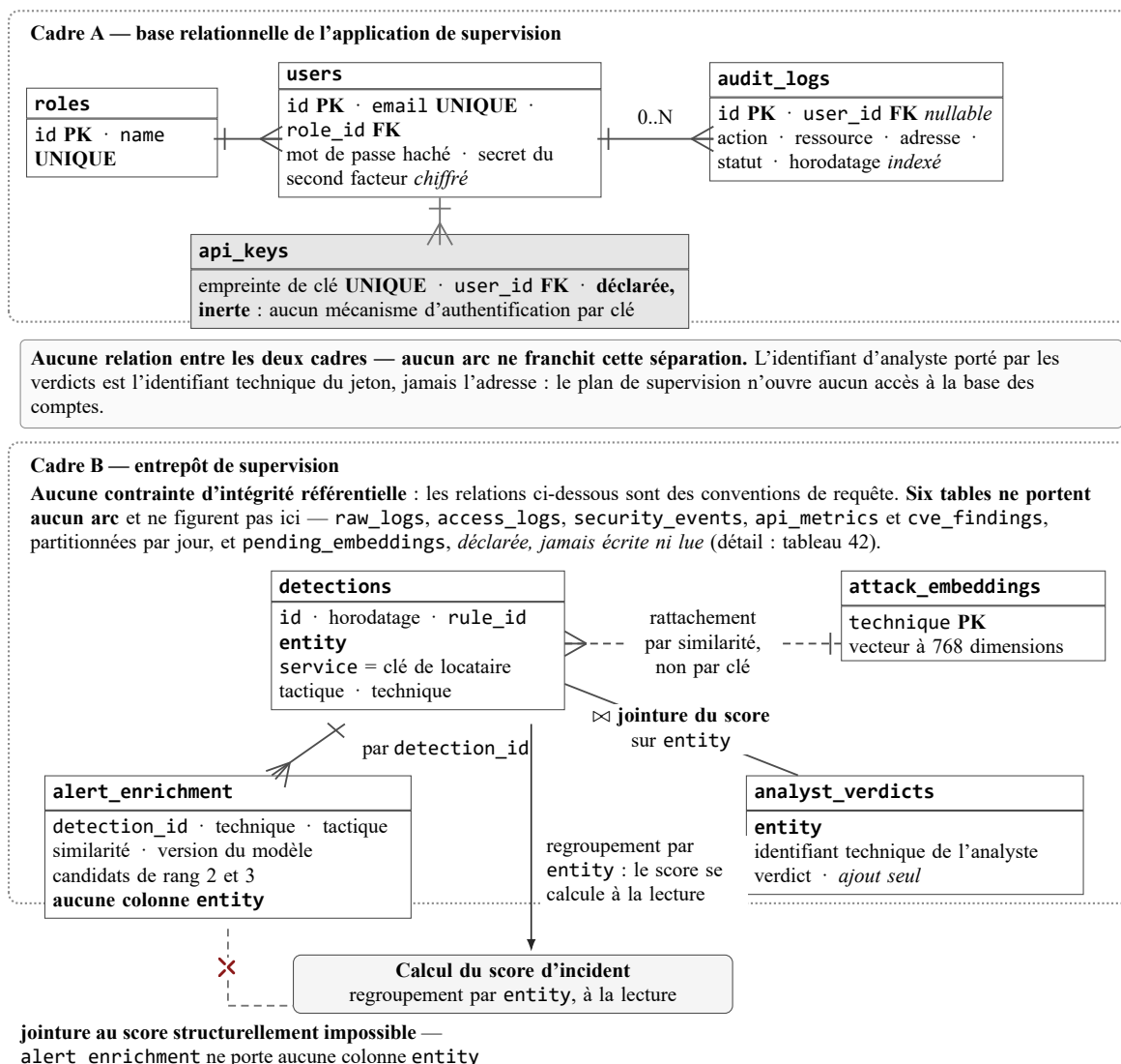
FIG. 15. Modèle de données des deux systèmes de stockage : ce que les clés permettent, et la jointure que leur absence interdit. L'impossibilité de corrélérer le rattachement sémantique au score d'incident est une propriété du schéma et non un choix d'algorithme — une colonne manquante suffit à l'expliquer — et les deux systèmes de stockage sont volontairement disjoints.
