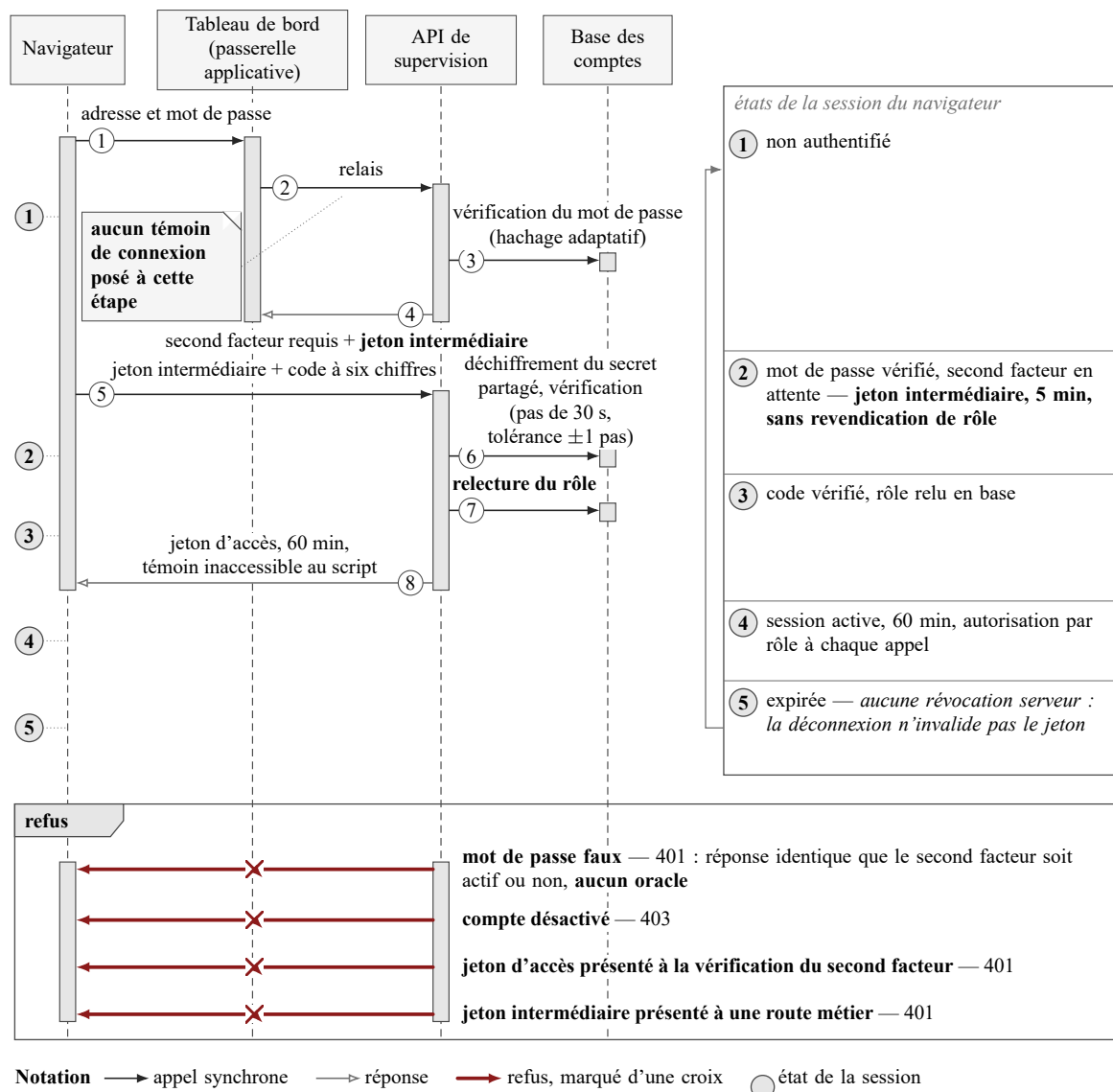
FIG. 19. Authentification à deux facteurs : cinq états de la session et le jeton intermédiaire qui ne porte aucun rôle. Entre le mot de passe et le code à usage unique, la session existe authentifiée mais non autorisée ; c'est la séparation des types de jeton — non le second facteur — qui interdit d'utiliser ce demi-passage.
