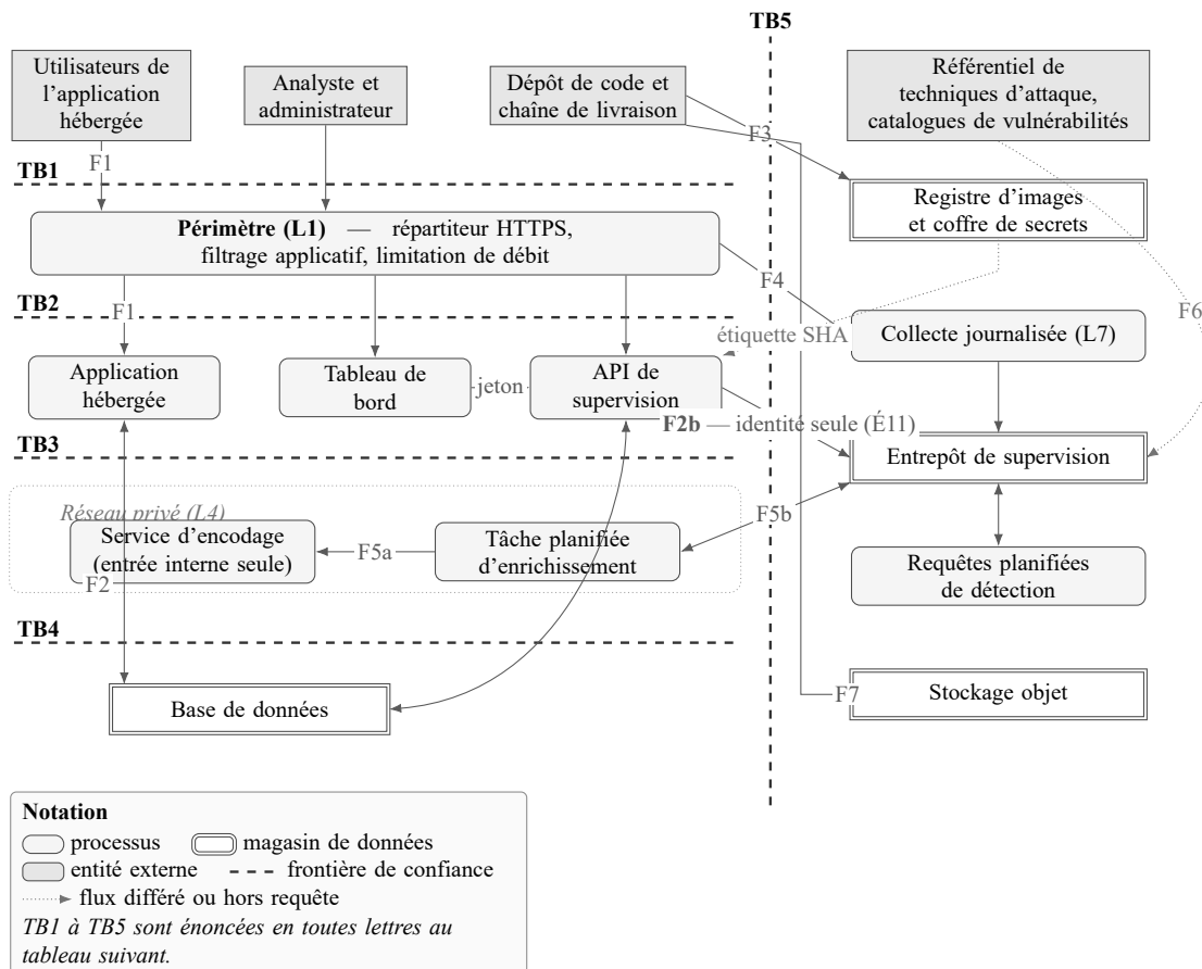
FIG. 8. Diagramme de flux de données du socle et ses cinq frontières de confiance. Les frontières TB1 à TB4 sont empilées et franchies par le réseau ; TB5 leur est orthogonale et n'est franchie que par l'identité. C'est cette frontière, sur laquelle aucun dispositif réseau ne peut s'interposer, que traversent douze des vingt-quatre scénarios opérationnels, dont six des huit scénarios de gravité critique.
