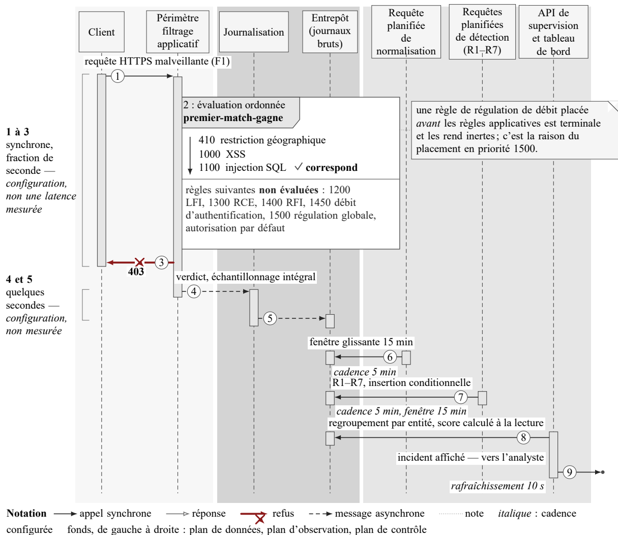
FIG. 16. Requête malveillante refusée au périmètre : ordre d'évaluation des règles et trajet de la preuve jusqu'à l'analyste. L'ordre est une propriété de sécurité — la première correspondance est terminale et les six règles suivantes ne sont jamais évaluées — et la preuve du refus met beaucoup plus de temps à atteindre l'analyste que le refus lui-même à être prononcé.
