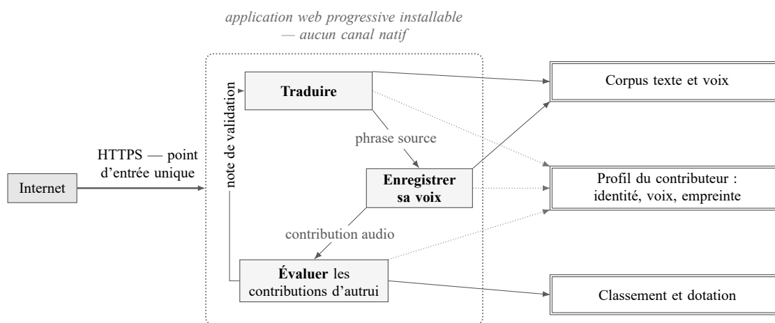
FIG. 3. Boucle fonctionnelle de l’application pilote et actifs produits. Chacun des trois temps produit un actif d’une nature différente — corpus, classement doté, profil de contributeur — alors que tous trois transitent par un seul point d’entrée HTTP.
